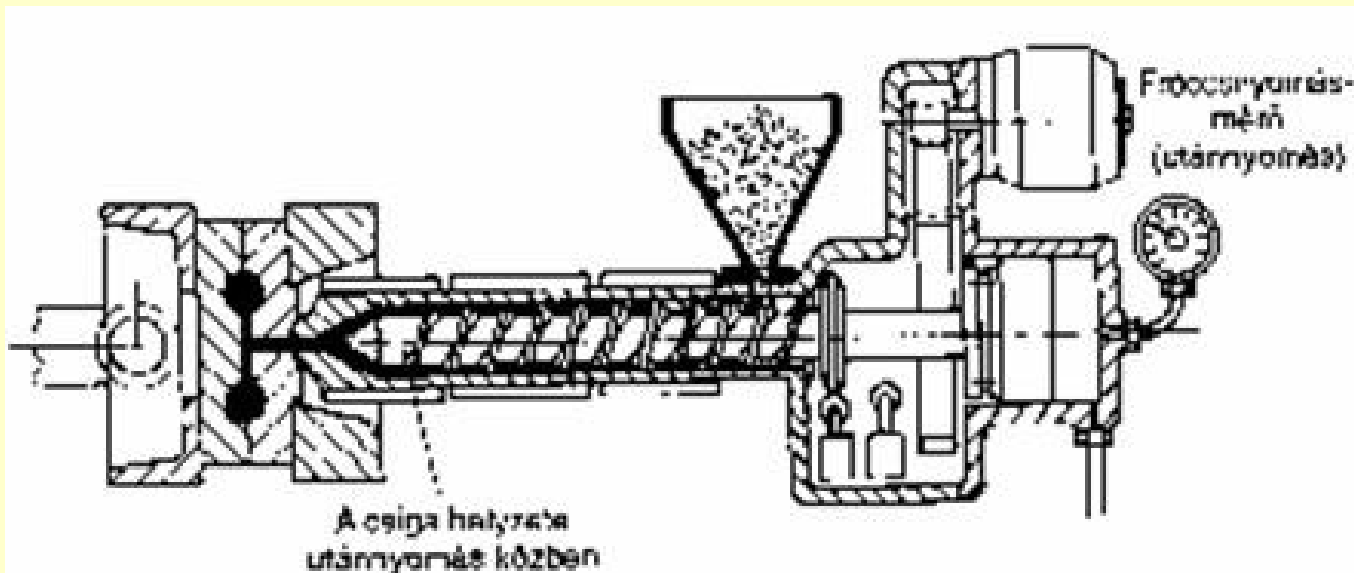
fröccsöntés
