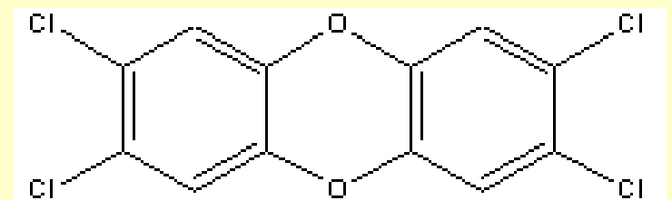
Tetrachlorodioxin
